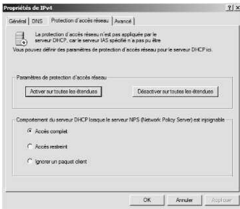
Figure 19-6 L'onglet Protection d'accès réseau contrôle les options de protection de DHCP.
