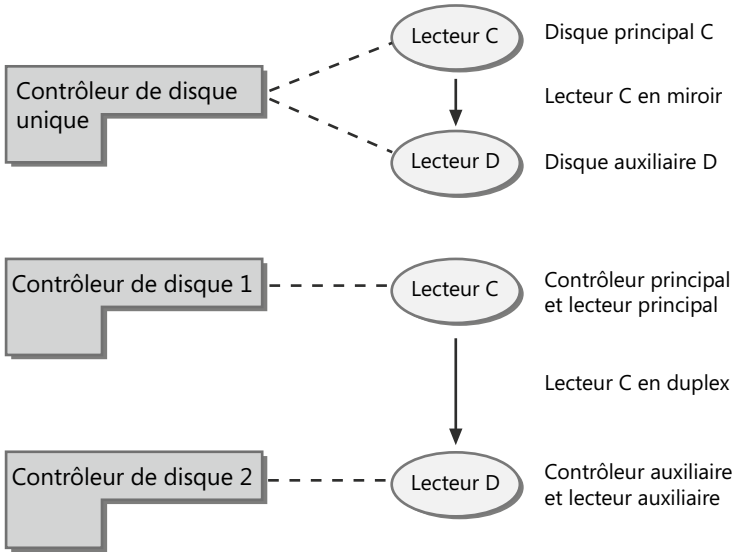
Figure 13-4 Alors que les disques en miroir n'utilisent habituellement qu'un contrôleur de disque pour créer un ensemble de données redondant, le duplexage de disques emploie deux contrôleurs.
