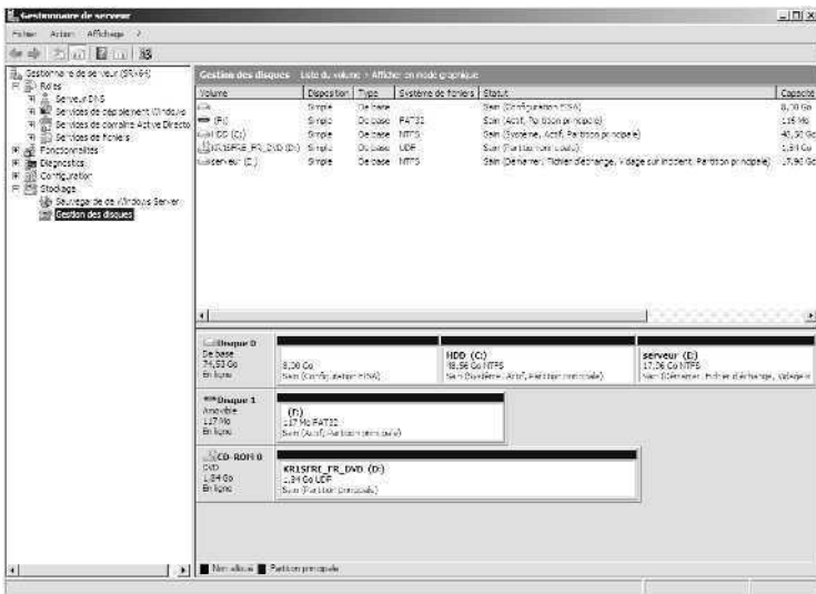
Figure 12-1 Dans Gestion des disques, par défaut, la partie supérieure propose une liste résumée détaillée de tous les lecteurs de l'ordinateur et la partie inférieure une représentation graphique de ces mêmes lecteurs.
