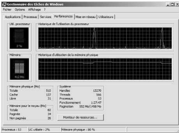
Figure 4-4 L'onglet Performances permet un contrôle rapide de l'utilisation des ressources du système.
