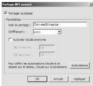
Figure 15-8 Avec le partage NFS, vous partagez des ressources entre des ordinateurs Windows et UNIX.
