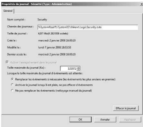
Figure 4-14 Paramétrez les options relatives aux journaux en fonction du niveau d'audit du système.
