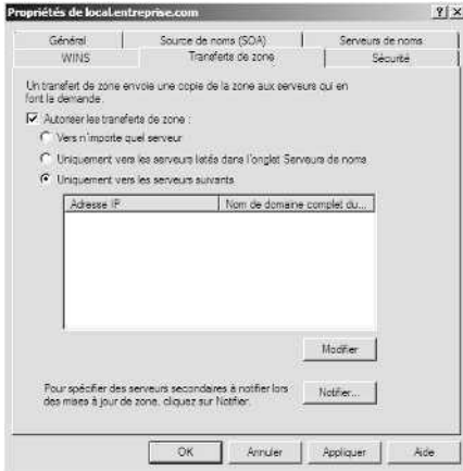
Figure 20-10 Servez-vous de l'onglet Transferts de zone pour autoriser les transferts vers tous les serveurs ou vers des serveurs spécifiques.
