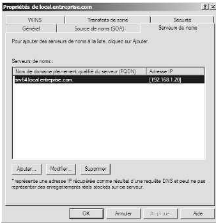
Figure 20-8 Configurez les serveurs de noms du domaine dans la boîte de dialogue Propriétés du domaine.
