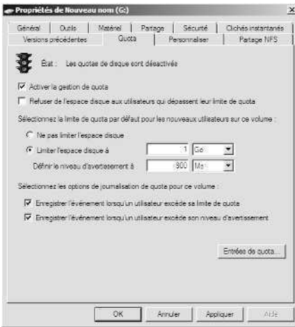
Figure 15-15 Après avoir activé la gestion des quotas, configurez une limite et un niveau d'avertissement pour tous les utilisateurs.
