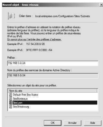
Figure 8-9 Créez le sous-réseau en saisissant le préfixe du réseau et en sélectionnant le site associé.
