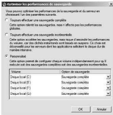
Figure 16-2 Configurez les paramètres sauvegarde par défaut.
