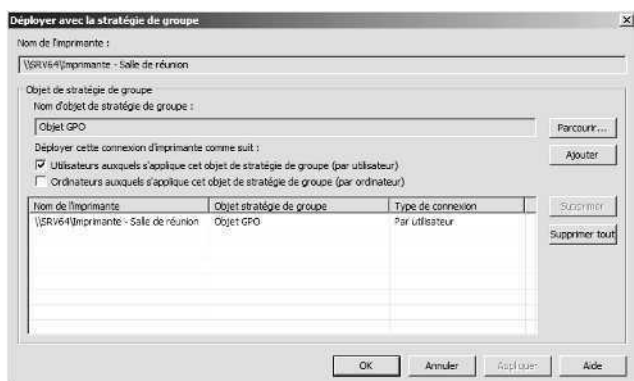
Figure 18-6 Sélectionnez le GPO à utiliser pour déployer la connexion d'imprimante.
