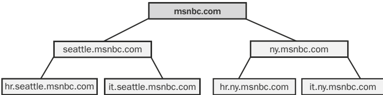
Figure 7-2 Les domaines d'une même arborescence partagent une structure de noms contiguë.
