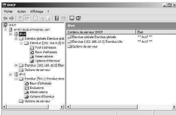
Figure 19-3 Utilisez la console DHCP pour créer et gérer les configurations de serveurs DHCP.
