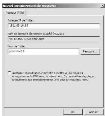
Figure 20-5 Si nécessaire, ajoutez des enregistrements PTR à tout moment à l'aide de la boîte de dialogue Nouvel enregistrement de ressource.
