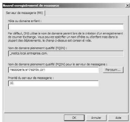
Figure 20-7 Les serveurs de messagerie dont la valeur préférentielle est la plus basse ont la plus grande priorité.
