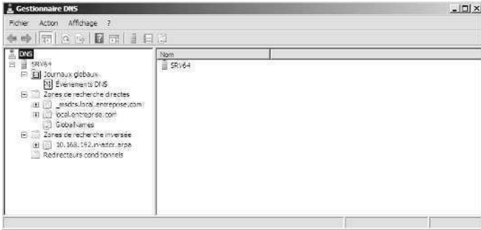
Figure 20-2 Les domaines et sous-réseaux se gèrent par l'intermédiaire des dossiers Zones de recherche directes et Zones de recherche inversée.
